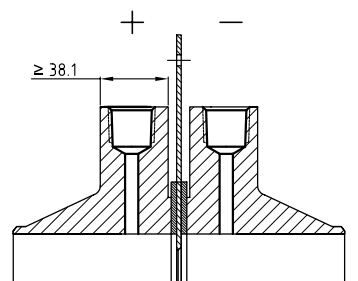
Flange tap
